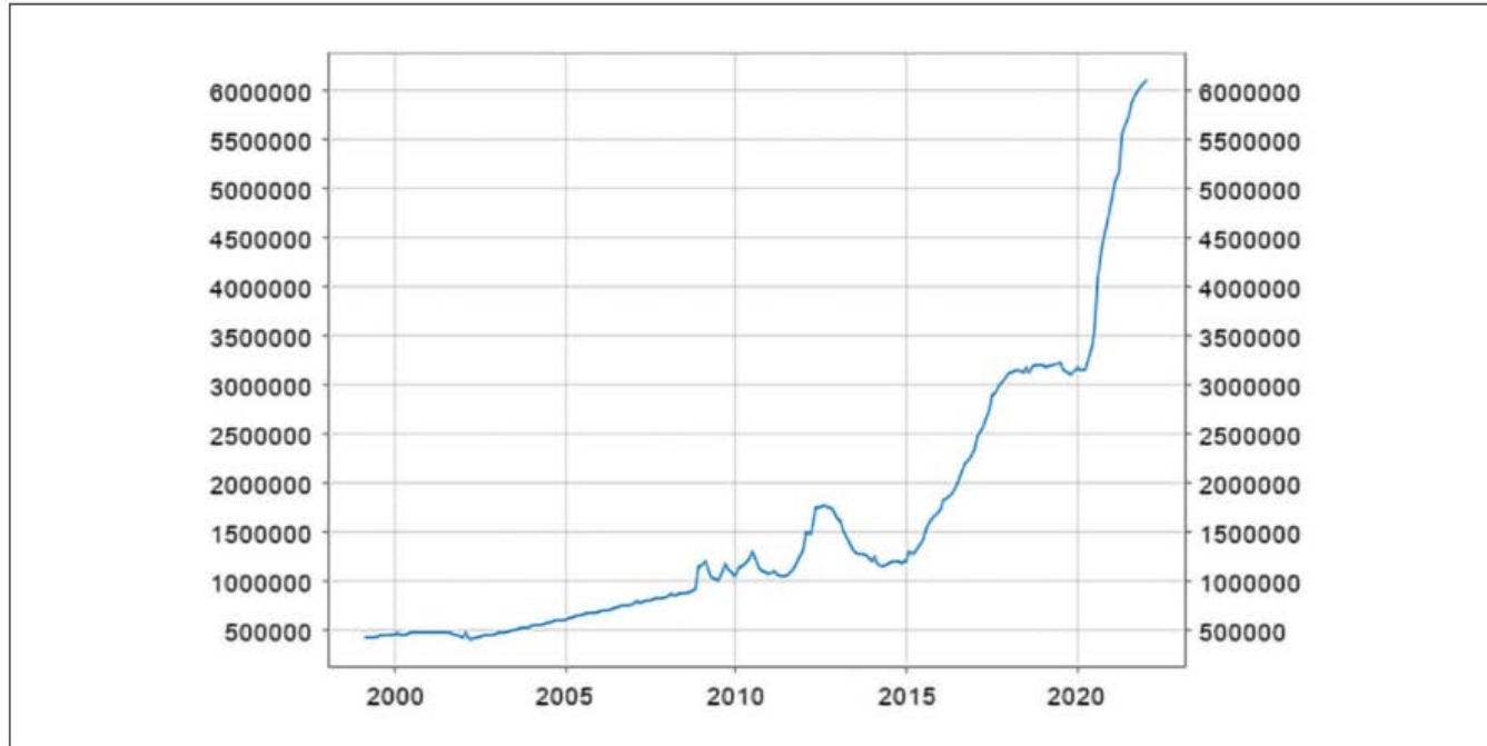
Figura 1 – Euro area: base monetaria 2000-2021
